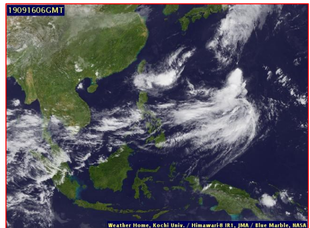
ภาพถ่ายดาวเทียม วันที่ ๑๖ ก.ย. ๒๕๖๒ เวลา ๑๓.๐๐ น.
