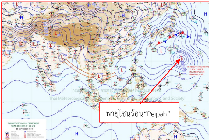
แผนที่อากาศ วันที่ ๑๖ ก.ย. ๒๕๖๒ เวลา ๐๗.๐๐ น.
